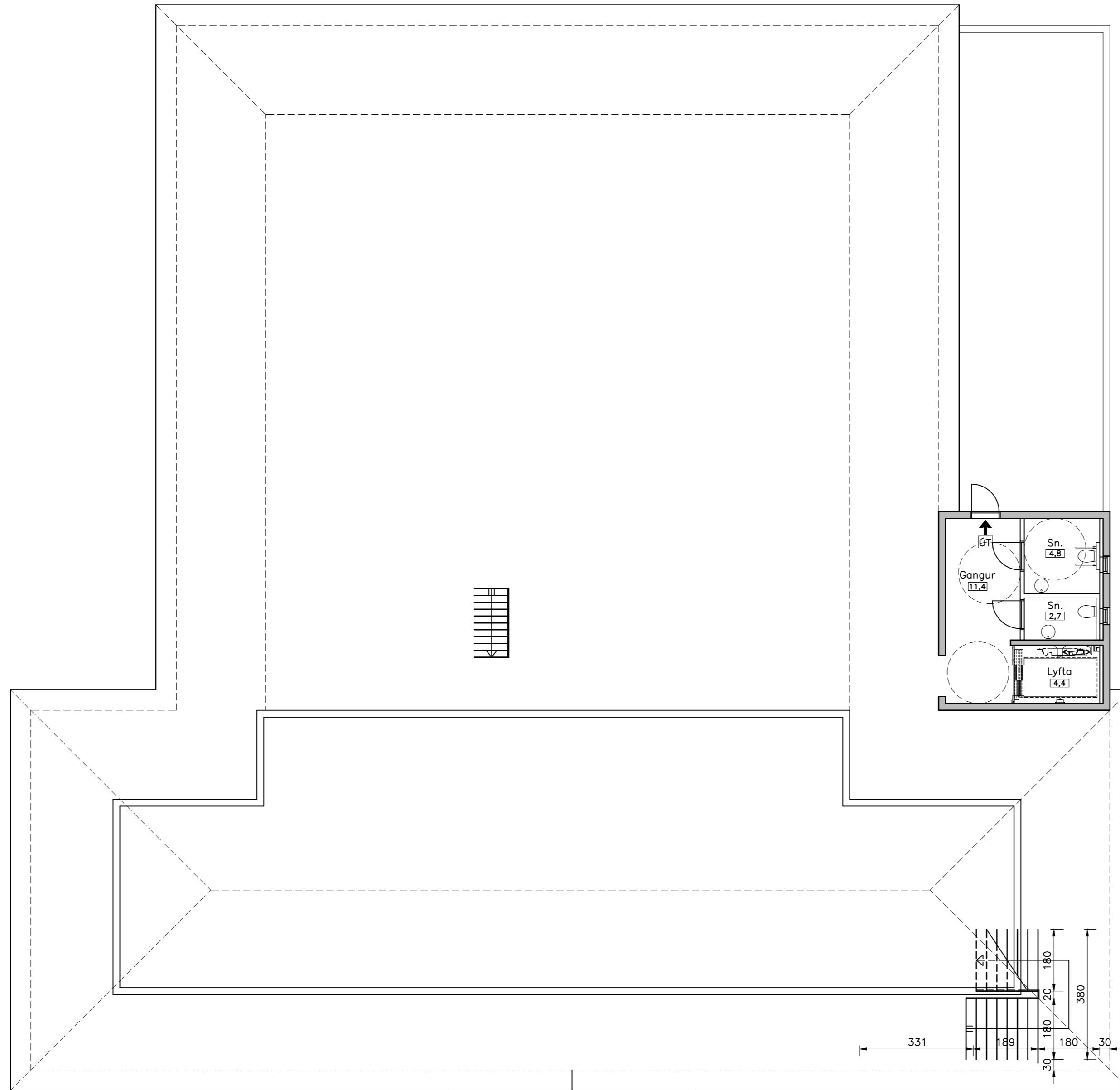
Grunnmynd rishæðar 1:100
